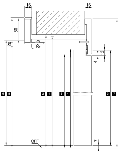
Vertikalschnitt
