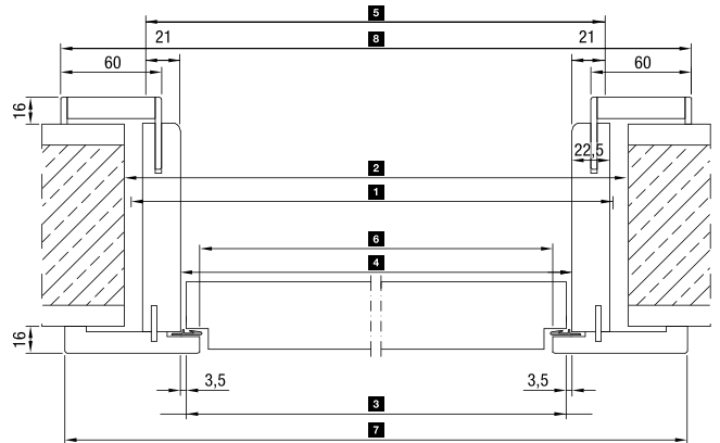
Horizontalschnitte
